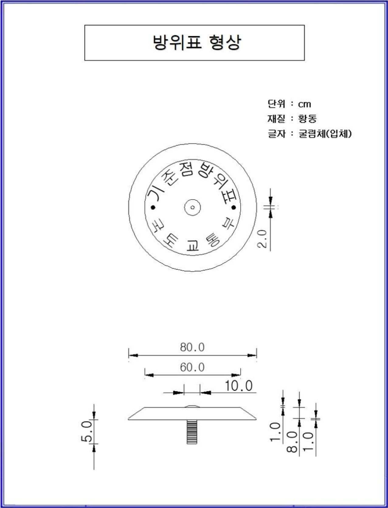
[별표 6-2] 방위표형상 (제17조제4항제4호 관련)
